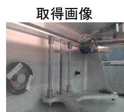
センター内の見える化(3Dプリンタの遠隔監視)
