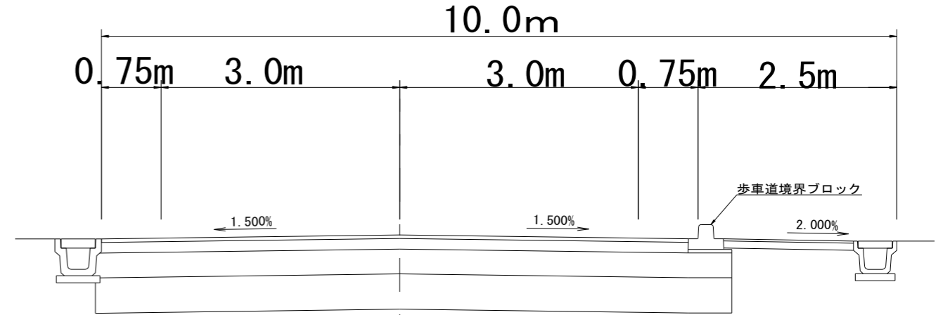
標準横断図
